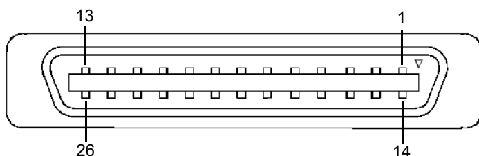
Fig. 1-11 Pinbelegung der Buchse IQ DATA
