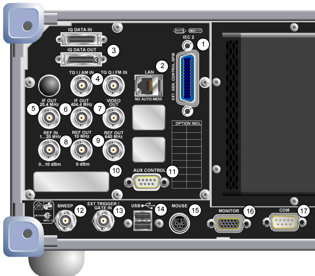
Fig. 1-5 Rückansicht
