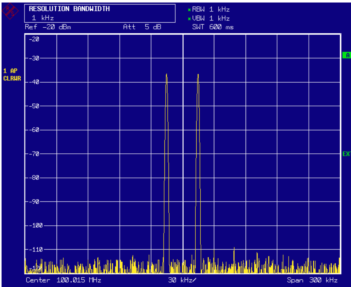
Fig. 5-8 Messung von zwei gleich großen HF-Sinussignalen mit einer Auflösesebandbreite (1 kHz), die deutlich kleiner ist als deren Frequenzabstand.
