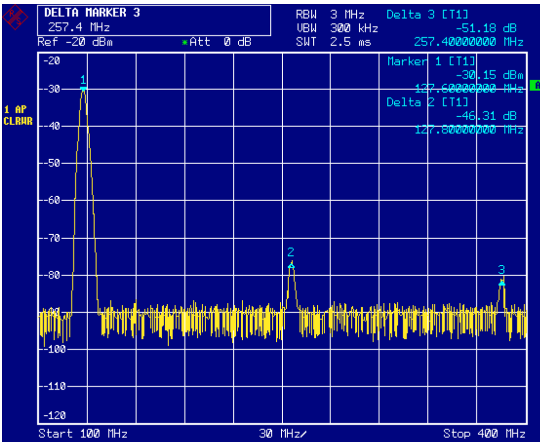
Fig. 5-2 Messung des Harmonischenabstandes des internen Referenzgenerators. Die Marker Delta 2 [T1] und Delta 3 [T1] zeigen den Abstand der ersten und zweiten Oberwelle zur Grundwelle an.
