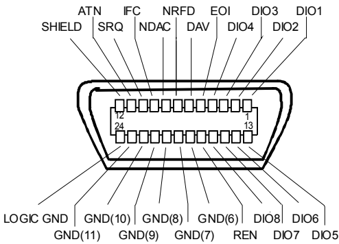
Fig. 1-9 Belegung der zweiten GPIB-Schnittstelle
